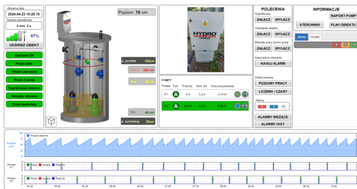
Panel synoptyczny przepompowni dostępny online
